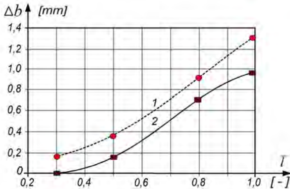
Rys. 12. Zmiana cięgiwy łopatki sprężarkowej
